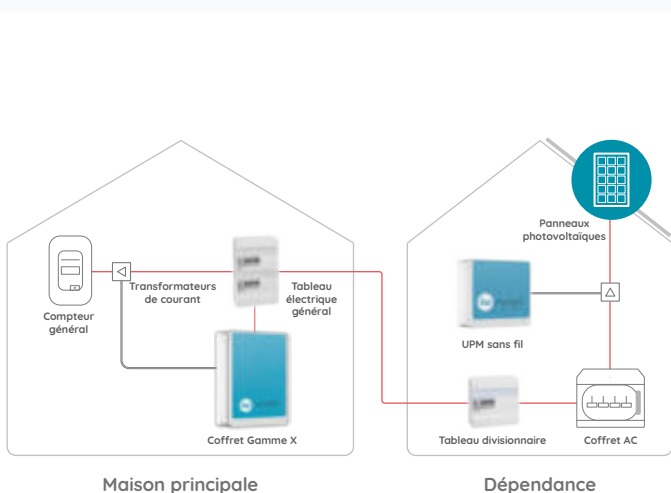
1 MESURE D'UNE PRODUCTION SOLAIRE DÉPORTÉE SUR UNE DÉPENDANCE
