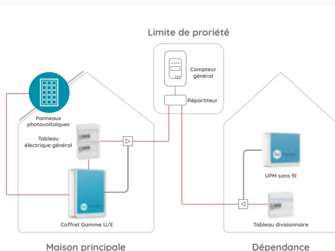
2 MESURE D'UNE CONSOMMATION SUR UNE DÉPENDANCE ÉLOIGNÉE
