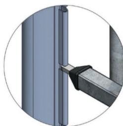
Pose avec les poteaux à encoches AXOR®, AXOR PLUS® ou AXIS®
