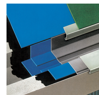
Détails d'étanchéité, chénaux : Colphène® 1500 + Colphène® 1560 Alu
