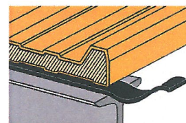
Figure 2 - Exemple de mise en oeuvre sur panne en couverture panneaux sandwiches
