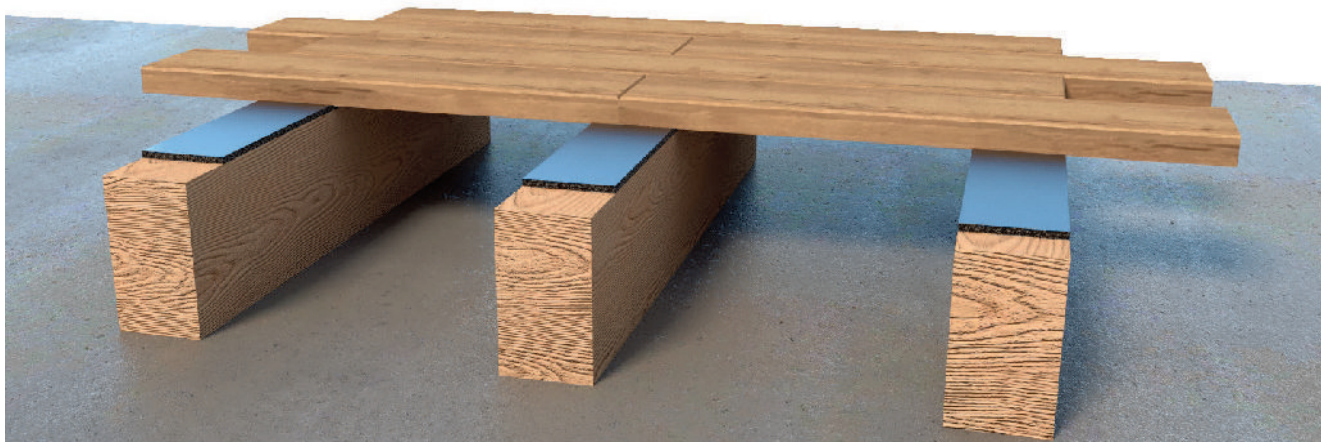
Pose du TRAMIBAND sur lambourde et plancher bois
