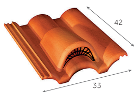
Tuile chatière grillagée (ouverture 18 cm 2 ) 5,7 kg/pièce
