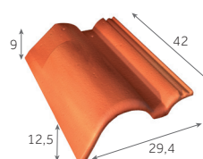
Tuile de rive ronde raccord gauche 4,4 kg/pièce
