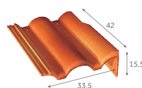
Tuile de rive universelle droite 3,2 au m 7,1 kg/pièce
