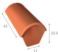
Faitière d'about de 42 (début)
