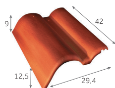
Rive ronde gauche 3,2 au m 4,3 kg/pièce
