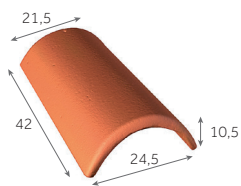
Faitière/arêtier de 42 à recouvrement
