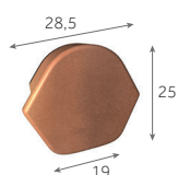
Fronton pour Faitière/arêtier de 42 à recouvrement
