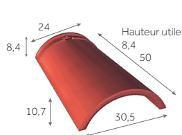
Faîtière/arêtier conique de 50 2,4 au m 4,3 kg/pièce
