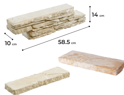
Blocs et couronnements Hadrien - Teinte Gironde
