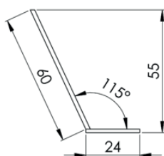
PEI60 Peigne d'avant-toit 60 mm
