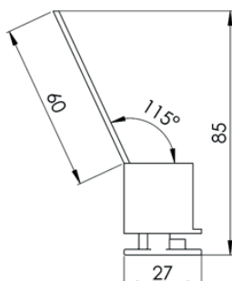
VL85 Liteau de ventilation avec peigne
