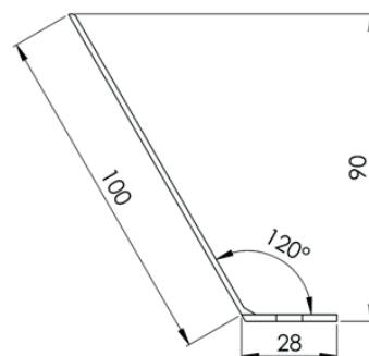
PEI100 Peigne d'avant-toit 100 mm
