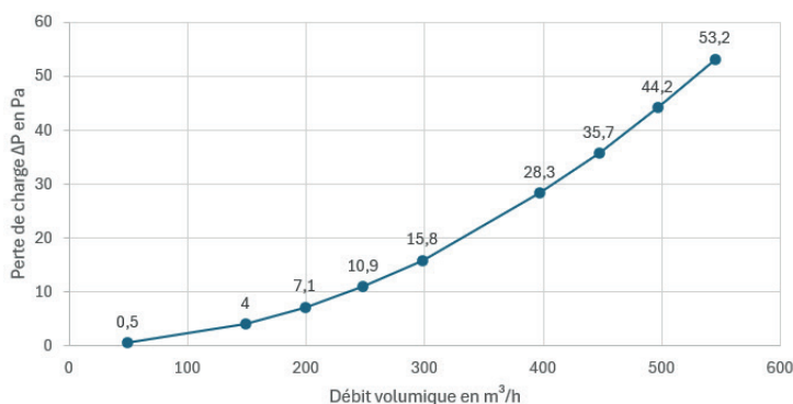
Pertes de charges chapeau NOTOS
