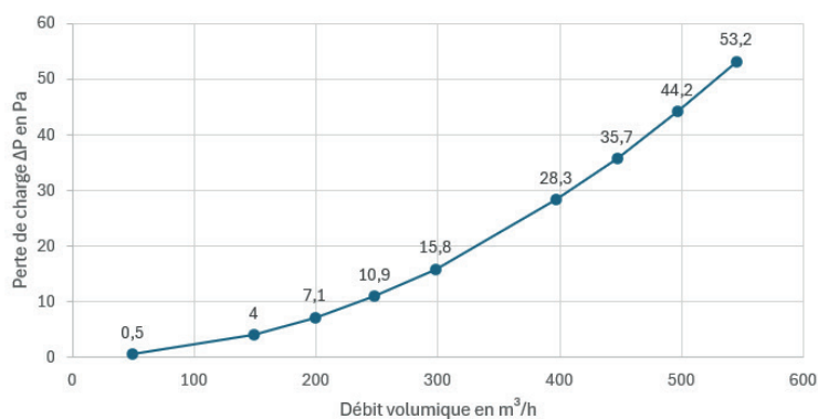
Pertes de charges chapeau NOTOS
